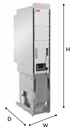
ACS880-04 frame D8T
